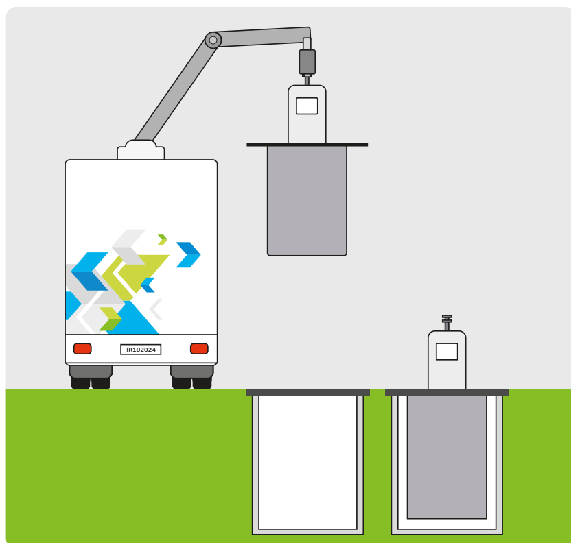
Tømming av nedgravd bunntømt container.
